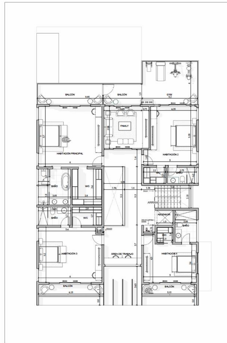
2 PLANTA ARQUITECTONICA DIMENSIONADA-NIVEL 2 1:75
