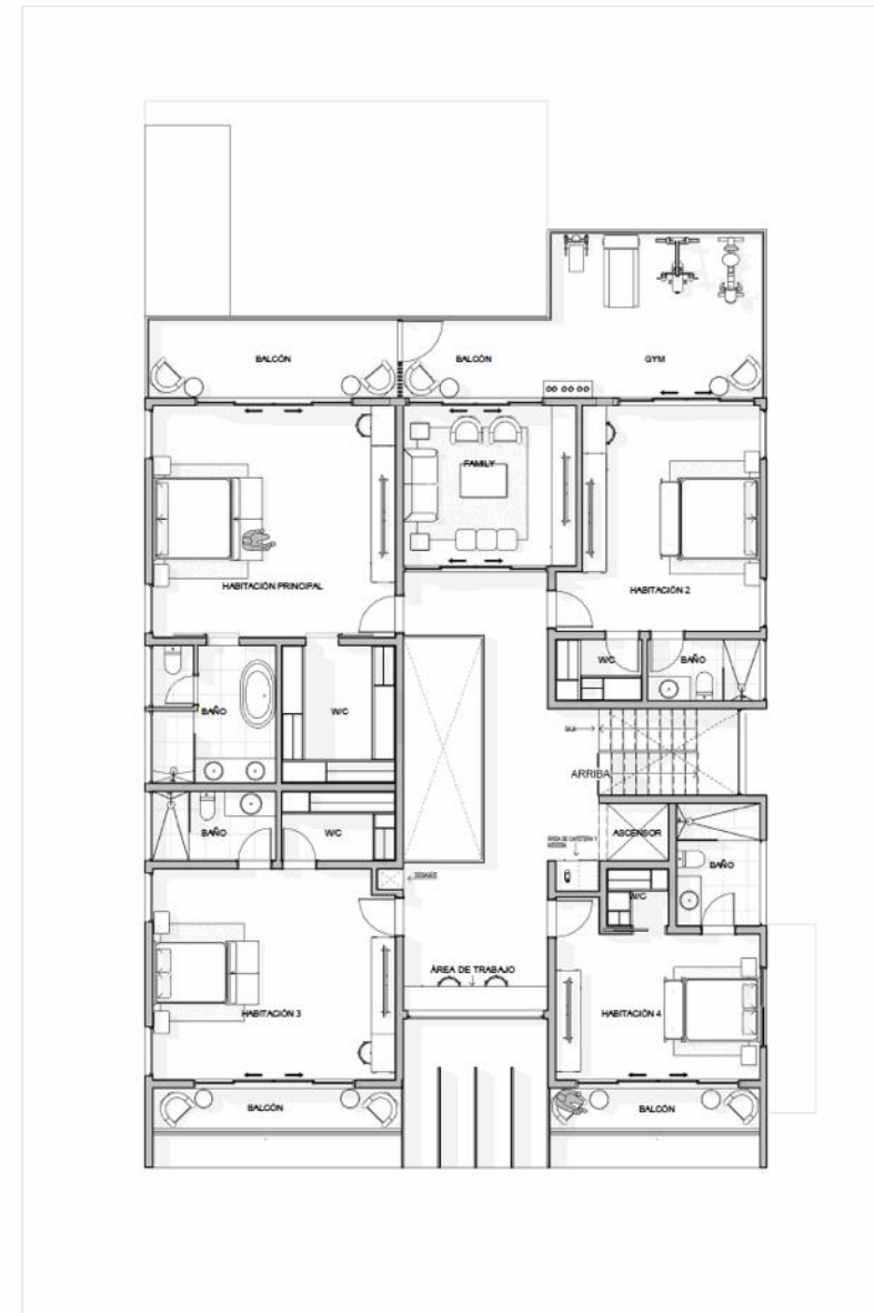
2 PLANTA ARQUITECTONICA-NIVEL 2 1:75
